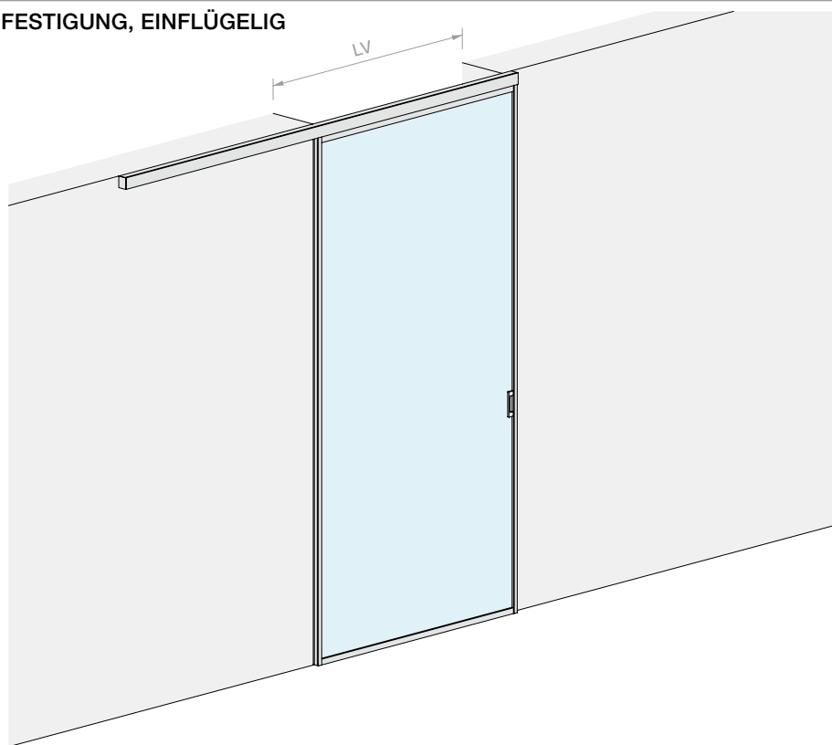
GLASTÜRFLÜGEL
