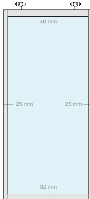
Türflügel einzelne Glasscheibe
