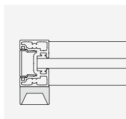
Art. MFM14025 verschraubt oder am Profil verklebt
