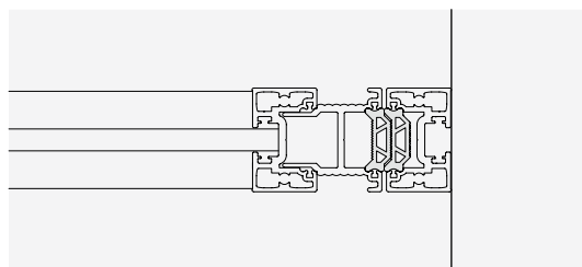
Dichtung beidseitig verwendbar
