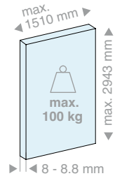
GLASTÜRFLÜGEL
