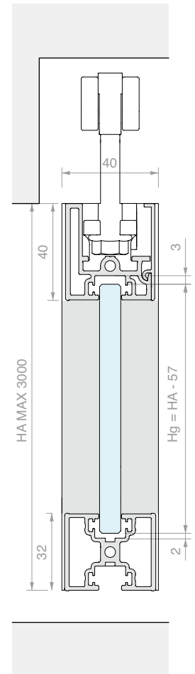
GLASTÜRFLÜGEL
