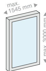
RAHMEN GLASTÜRFLÜGEL
