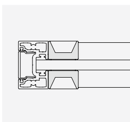
Art. MFM14025 am Glas verklebt
