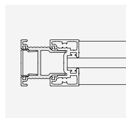
Art. LMC0038 extrudiert auf ganzer Höhe verschraubt, mit oder ohne Dichtung
