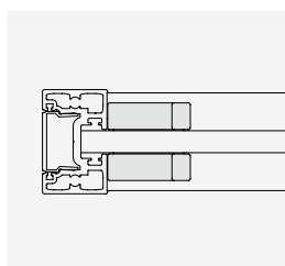
Art. HAND32140VHB am Glas verklebt
