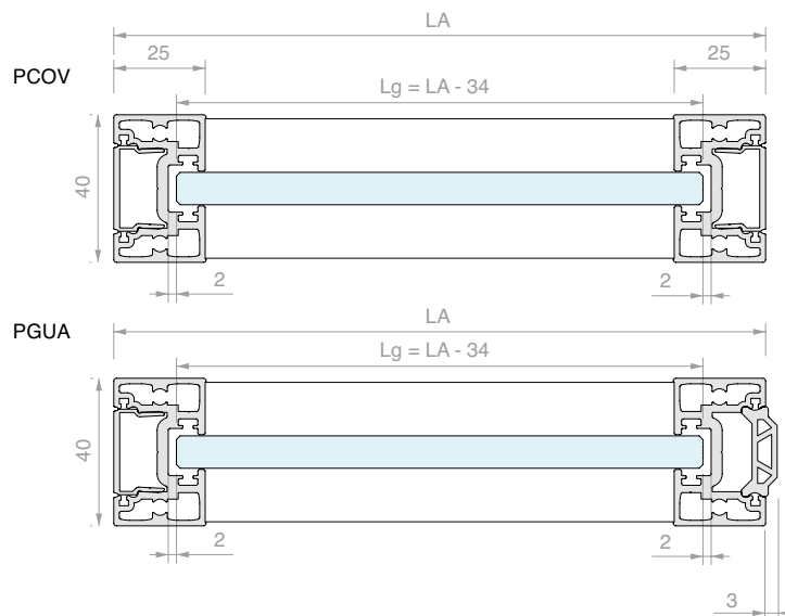
RAHMEN GLASTÜRFLÜGEL
