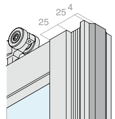
mit Griff auf ganzer Höhe und Anschlagdichtung
